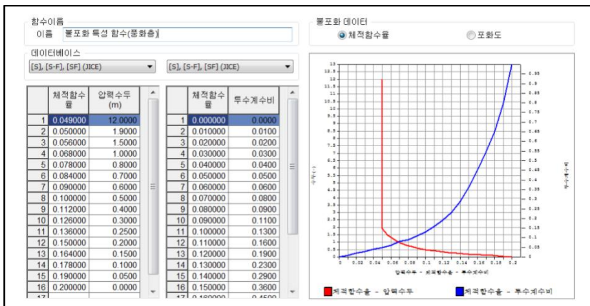
【그림 17.15】 압력수두-채적함수(포화도)-투수계수비 함수
