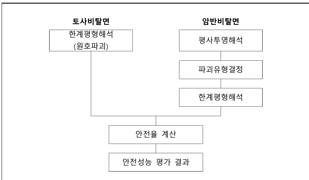
【그림 17.5】 구조안전성능 평가과정
