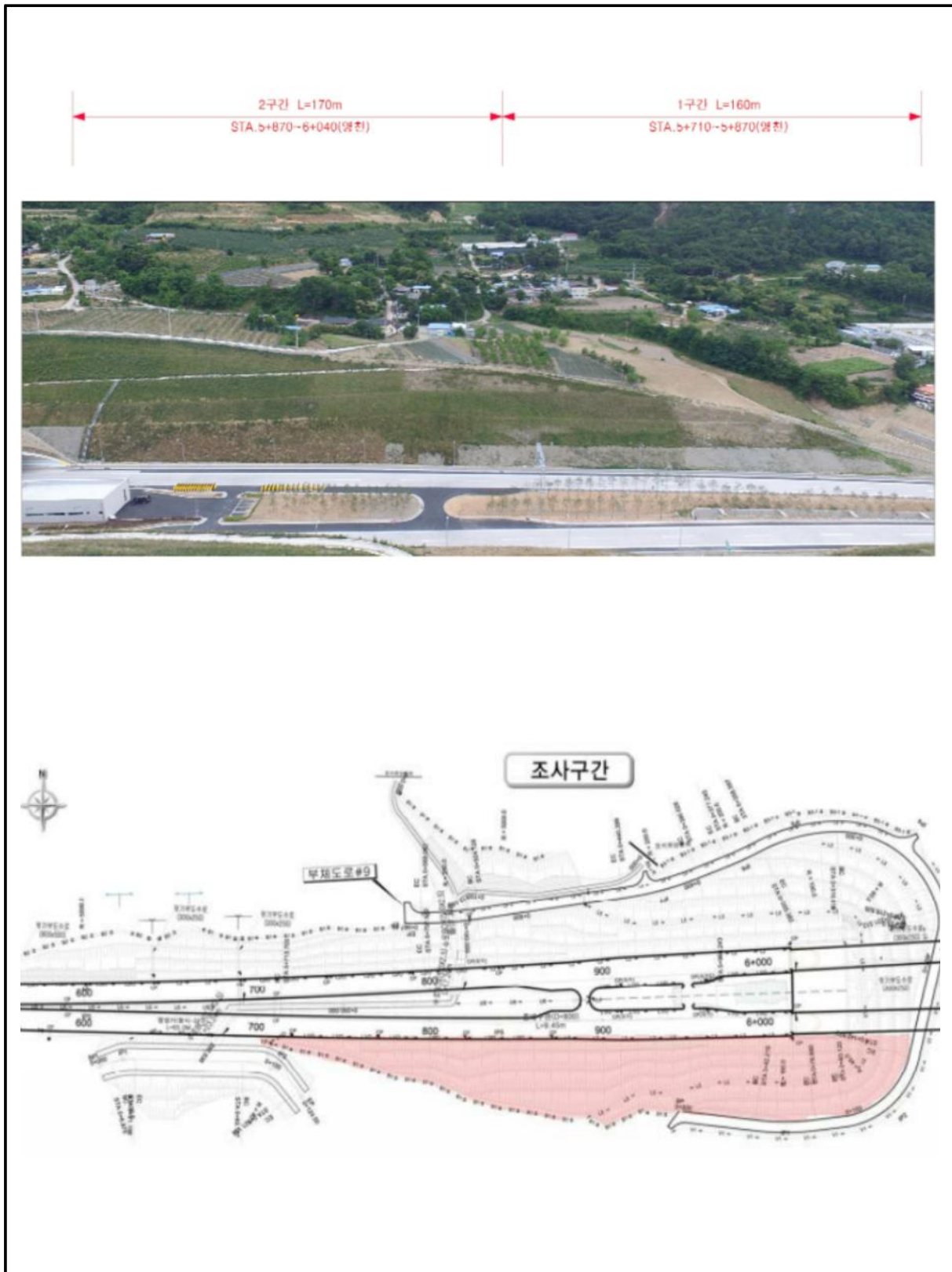
【그림 17.14】 영천절토17 검토대상 비탈면구간
